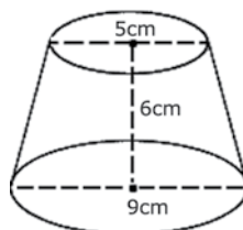
Διαστάσεις κώνων
